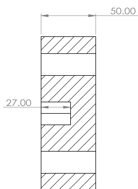
断面図 B-B
