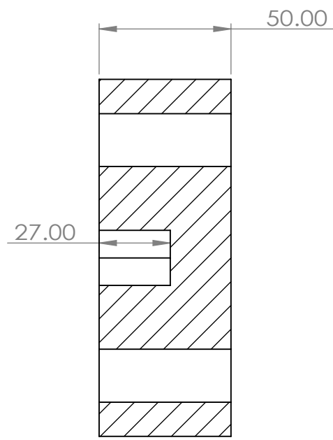
断面図 B-B
