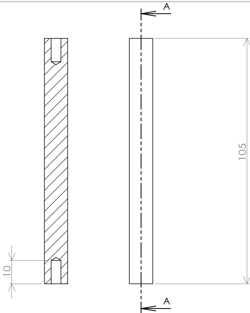
断面図 A-A
