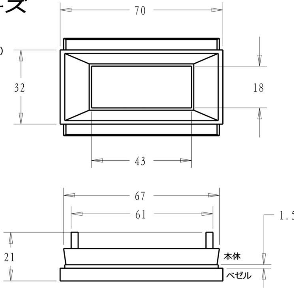
パネル加工参考図面(1)
